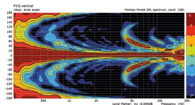
Vertikales Richtverhalten
