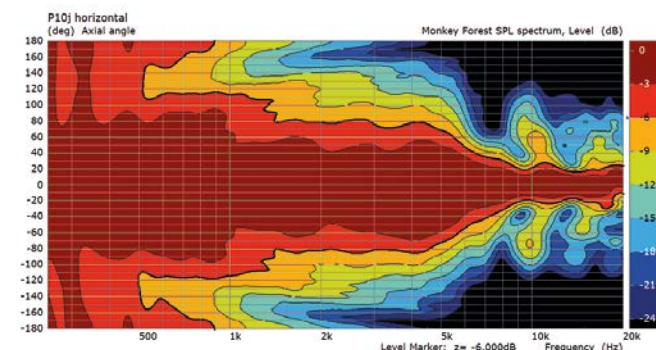
Horizontales Richtverhalten
