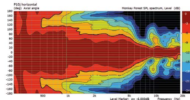
Horizontales Richtverhalten
