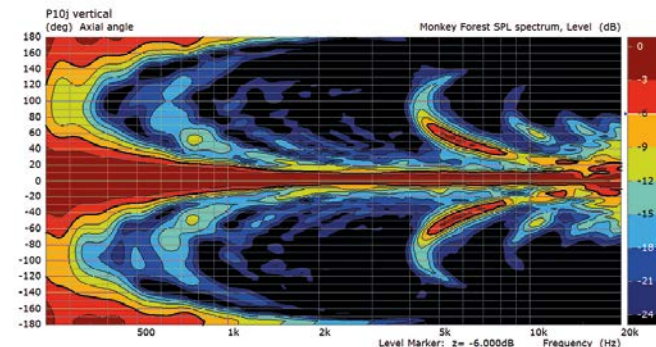
Vertikales Richtverhalten
