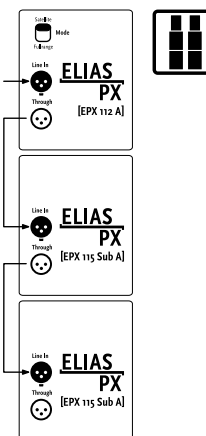
Anschluss-Schema Extension-Setup
