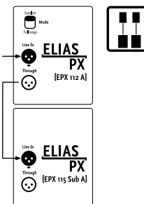
Anschluss-Schema Standard-System
