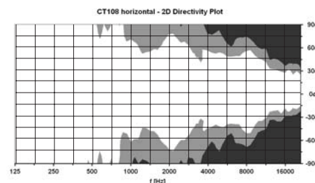
Abbildung 3: Abstrahlverhalten CT 108 horizontal
